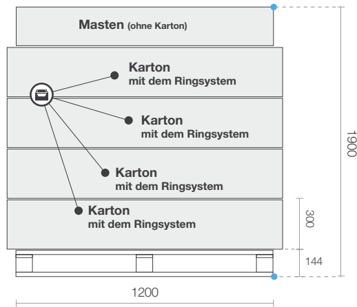
A Seitenansicht
