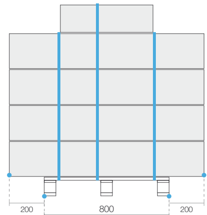
B Vorderansicht
